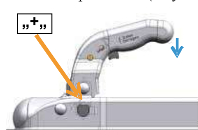
3. Kapcsolódva (lenyomva)
