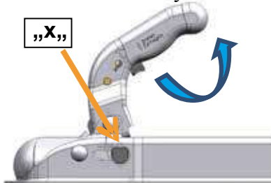
2. Nyitott
